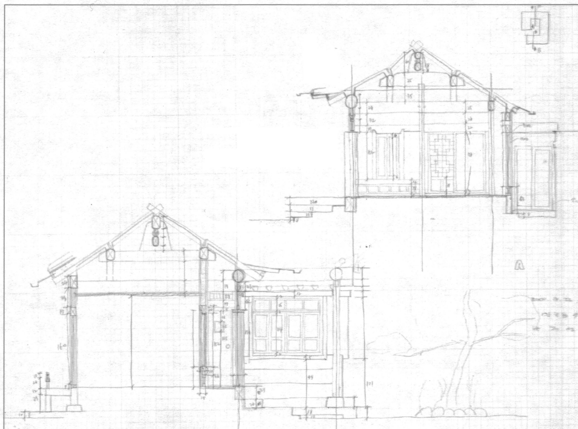
실측도면(단면)
