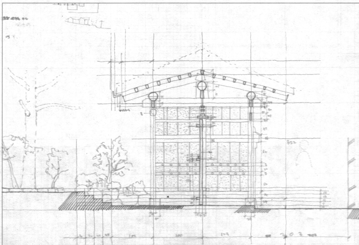
실측도면(대문)
