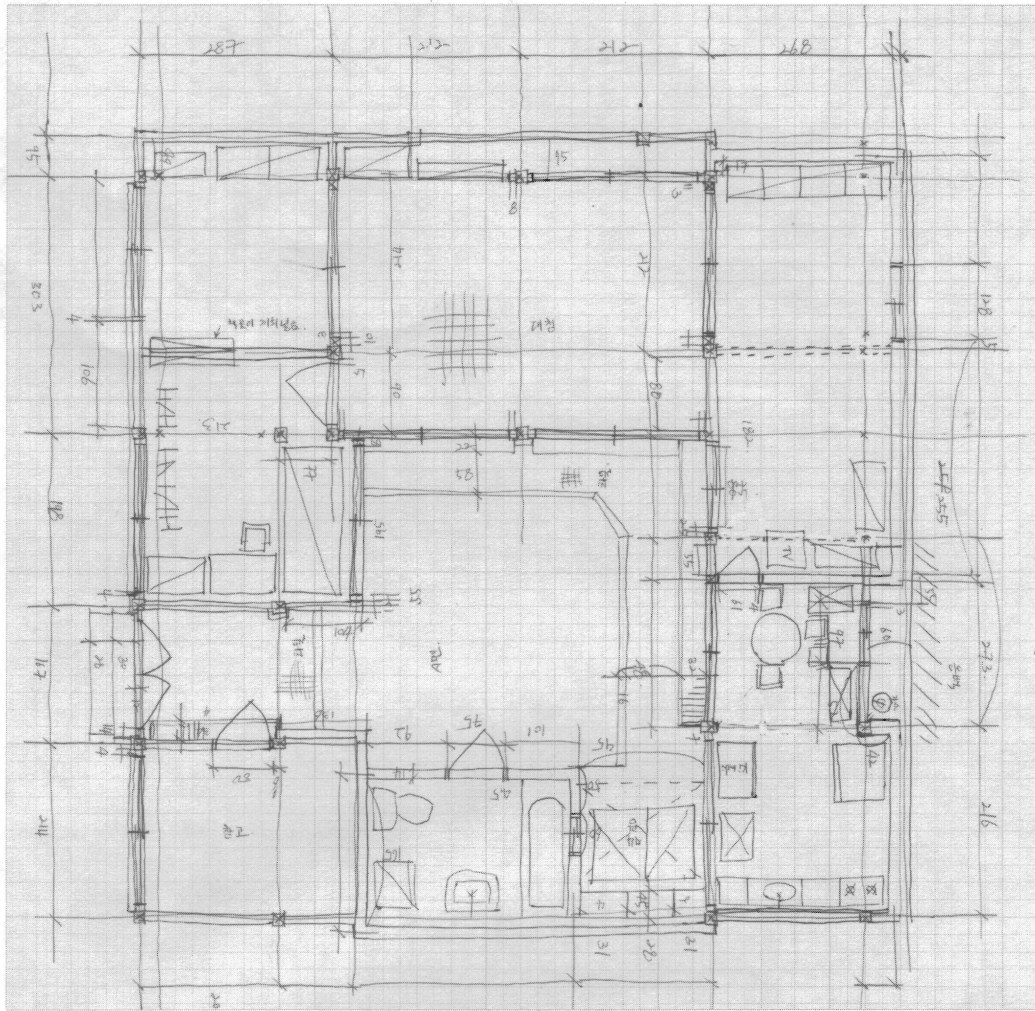
실측도면(평면)
