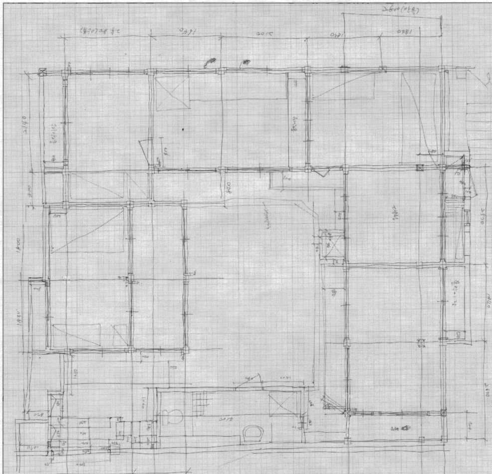
실측도면(평면)
