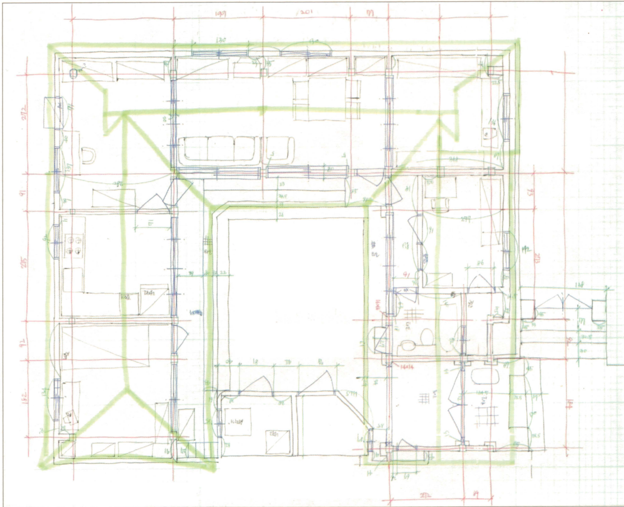
실측도면(평면)
