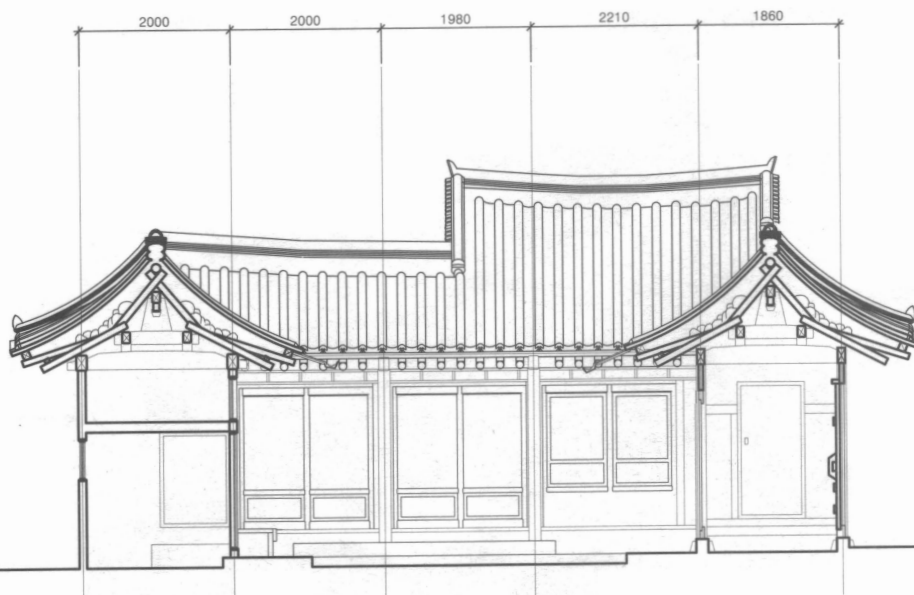
A-A' 단면도
