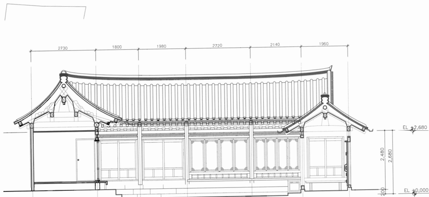
A-A' 단면도
