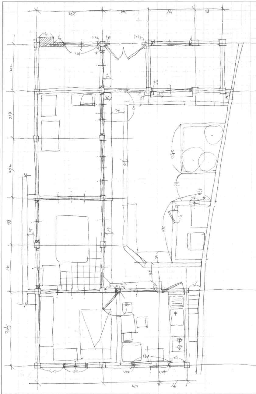
실측도면(평면)
