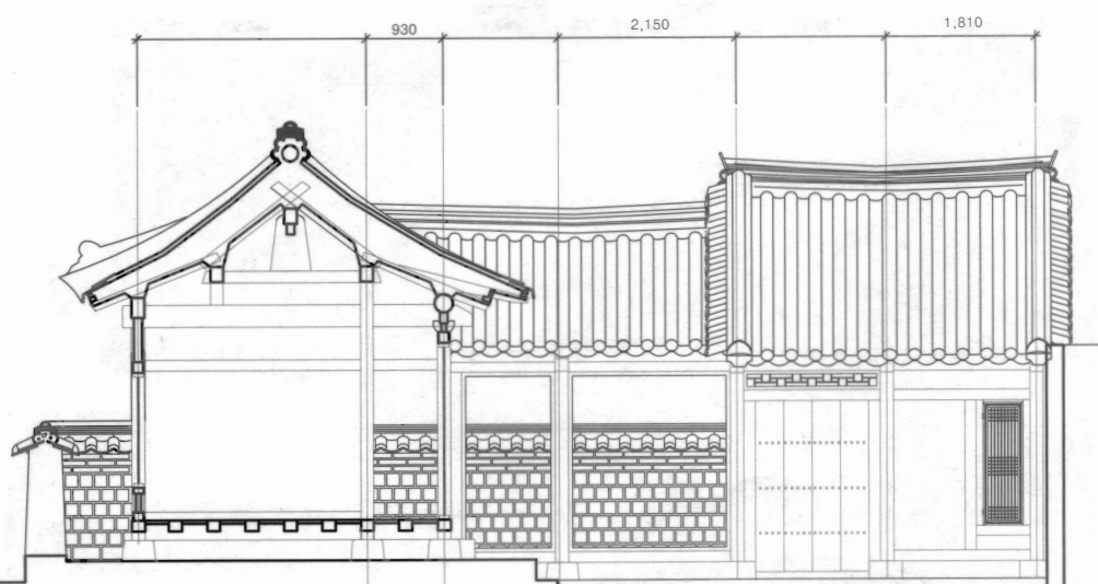
A-A' 단면도
