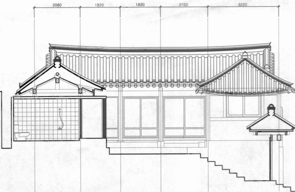
A-A' 단면도
