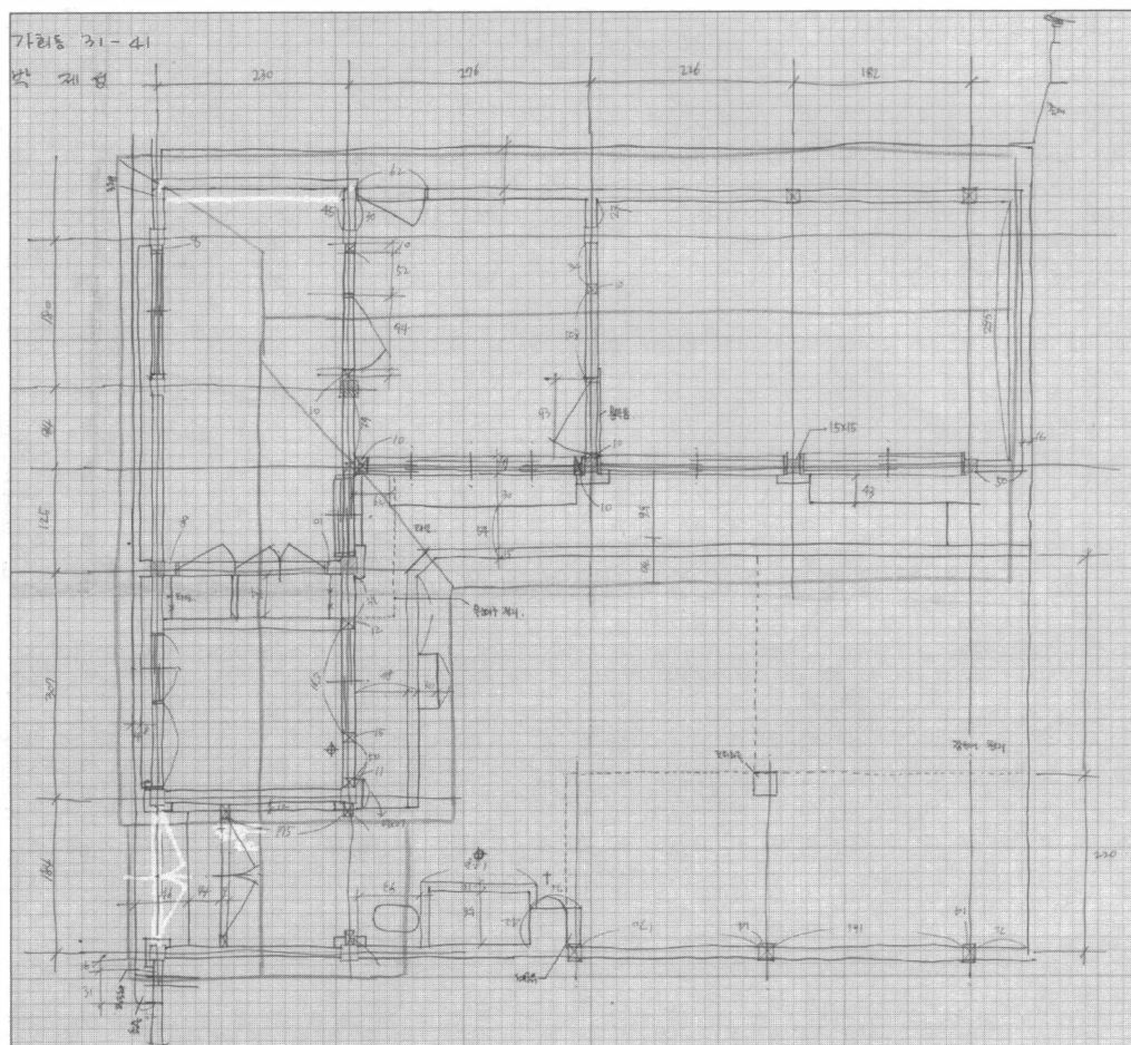
실측도면(평면)
