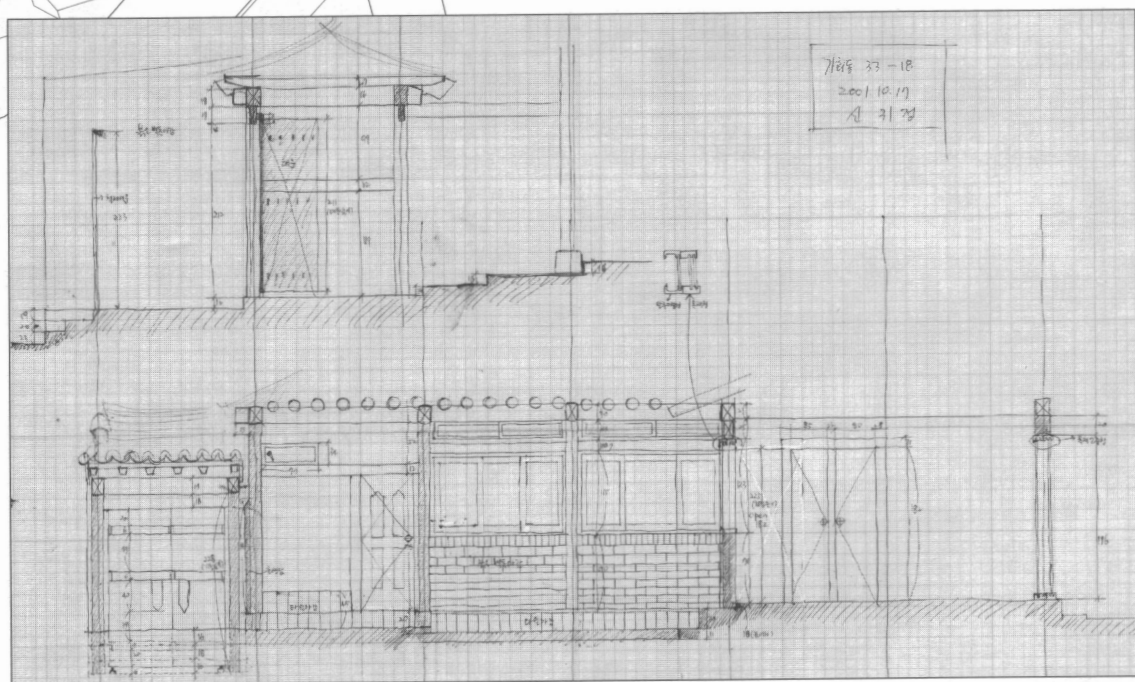
실측도면(단면)
