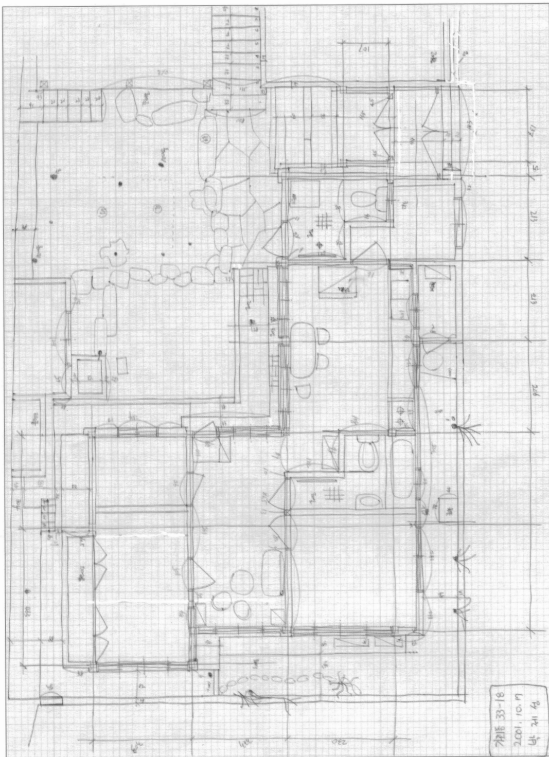
실측도면(평면)
