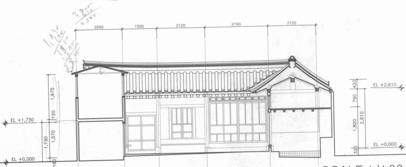
A-A' 단면도
