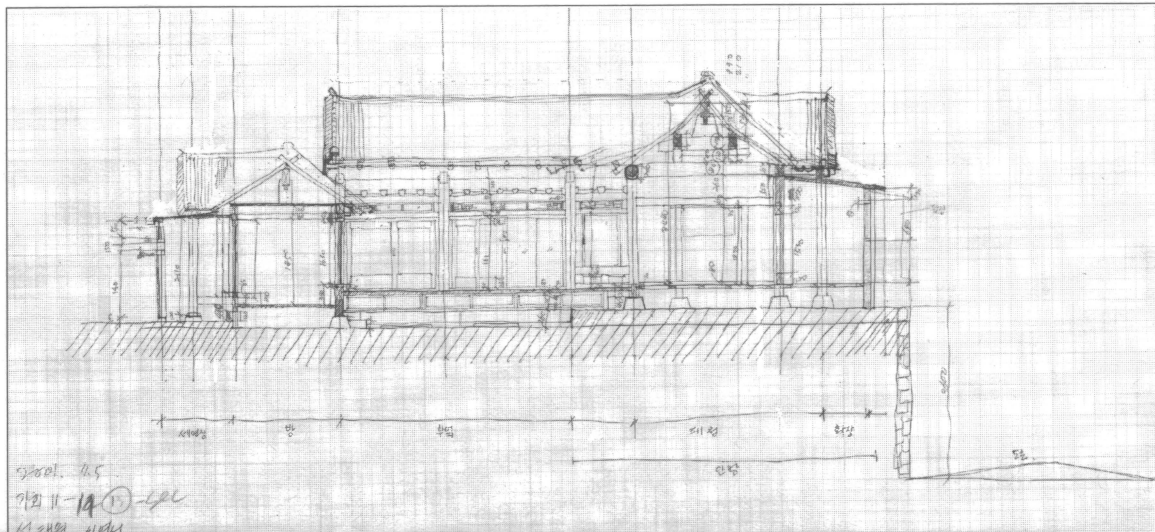
실측도면(단면)
