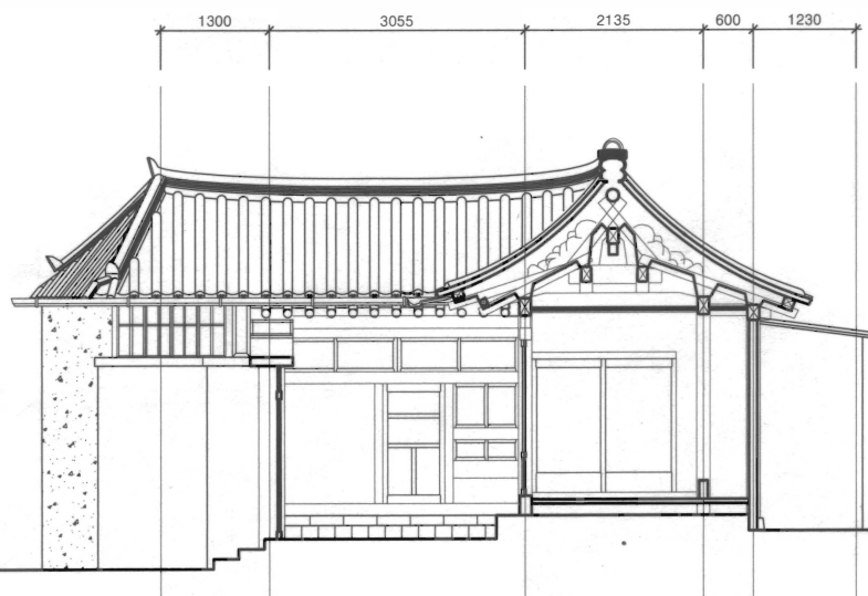
A-A' 단면도
