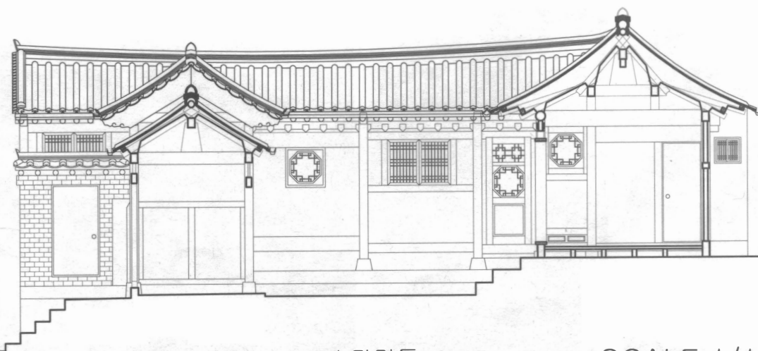
A-A' 단면도
