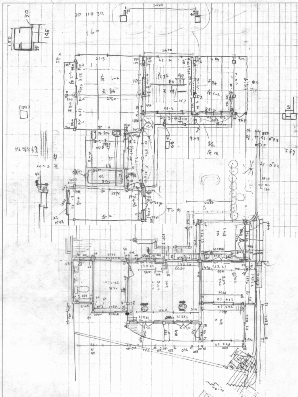
실측도면(평면)
