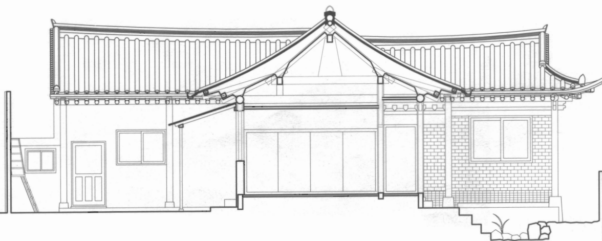
A-A' 단면도
