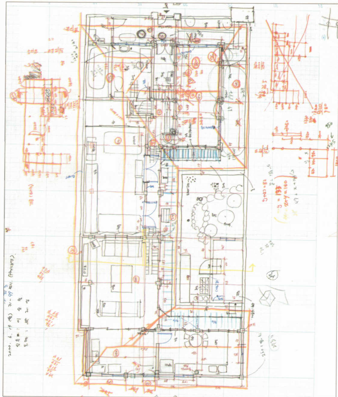
실측도면(평면)
