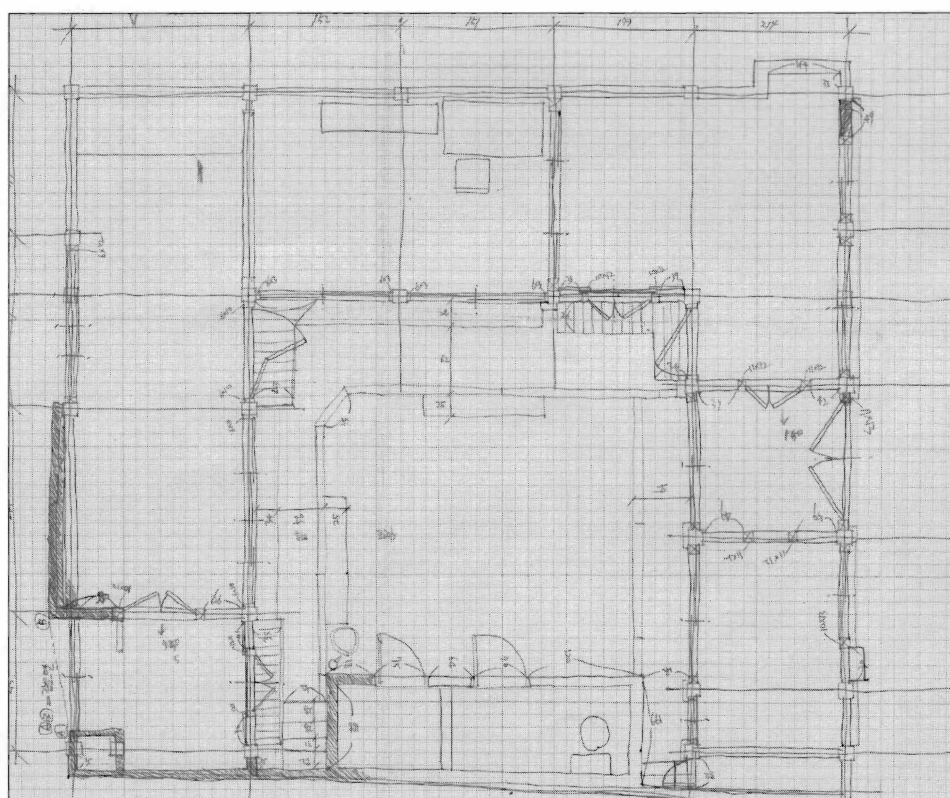
실측도면(평면)
