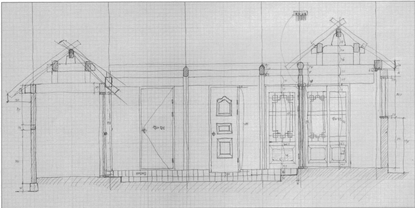
실측도면(단면)
