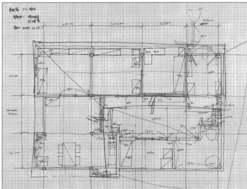
실측도면(평면)
